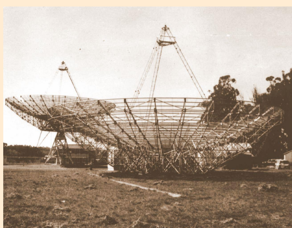
Construcción de las costillas de la Antena II
