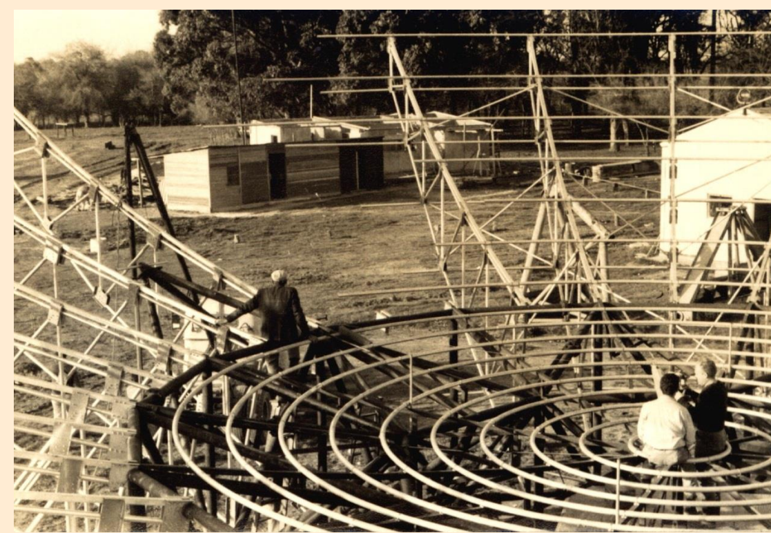
Ajuste de los anillos con teodolito
