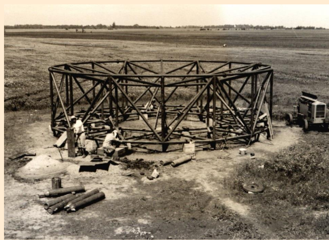
Construcción de la base de la Antena I
