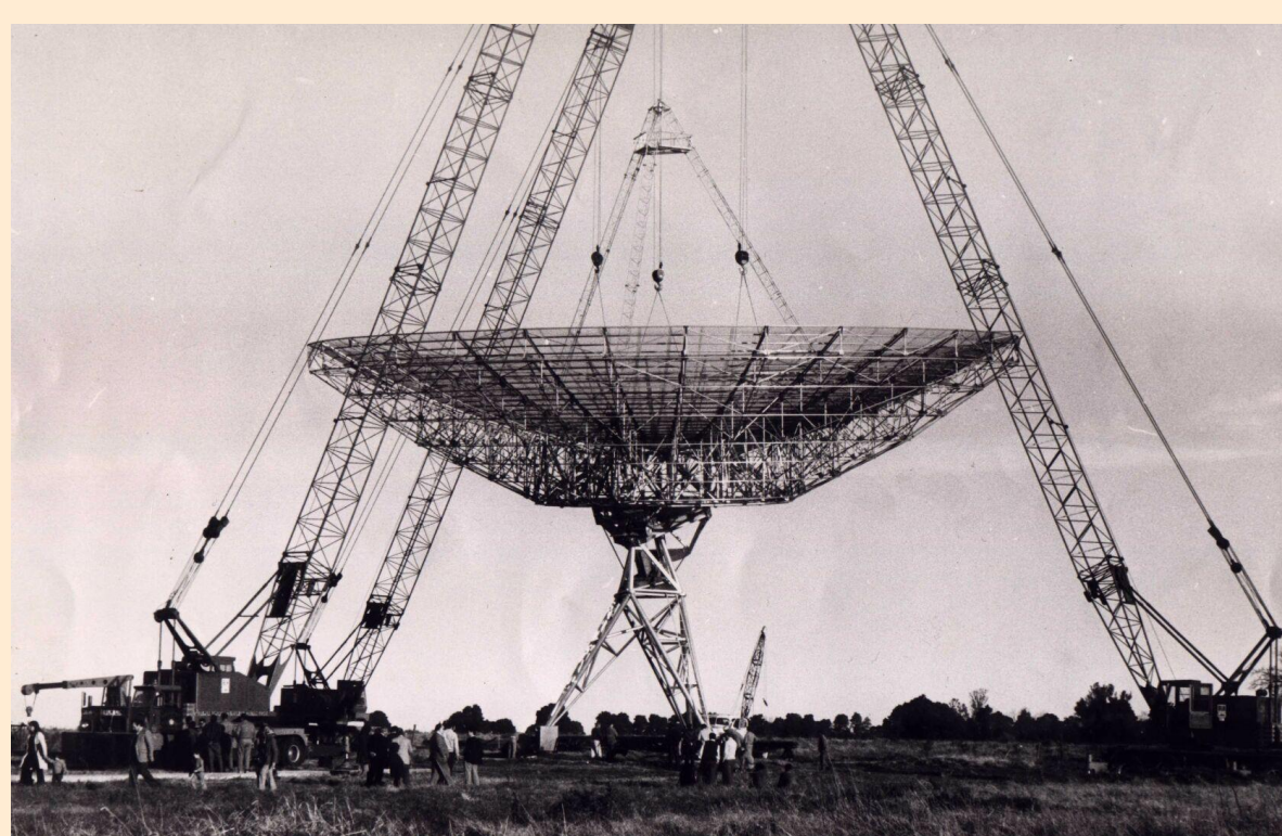
Montaje de la Antena II sobre la base
