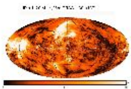
Relevamiento de todo el cielo en 1420 MHz de la intensidad polarizada (IP) resultante de la combinación del ambos relevamientos
